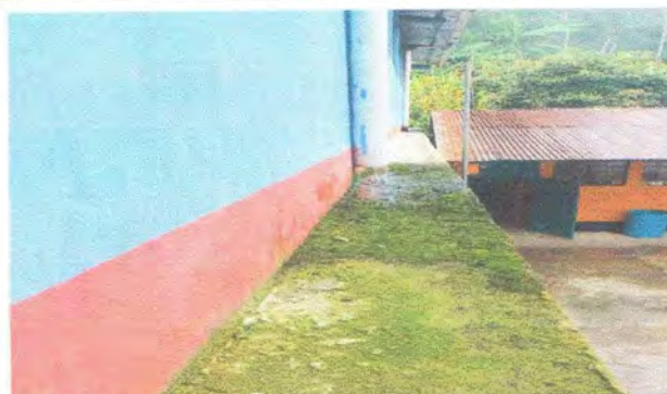
Foto 2: Reparacion de bajada de agua pluvial, tubo PVC 3"
